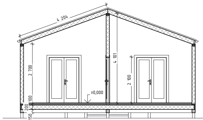
Разрез 1-1
