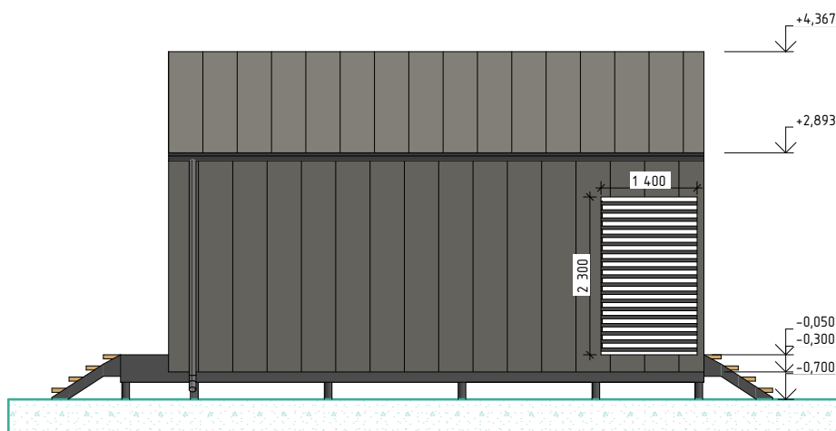
Фасад А-Д
